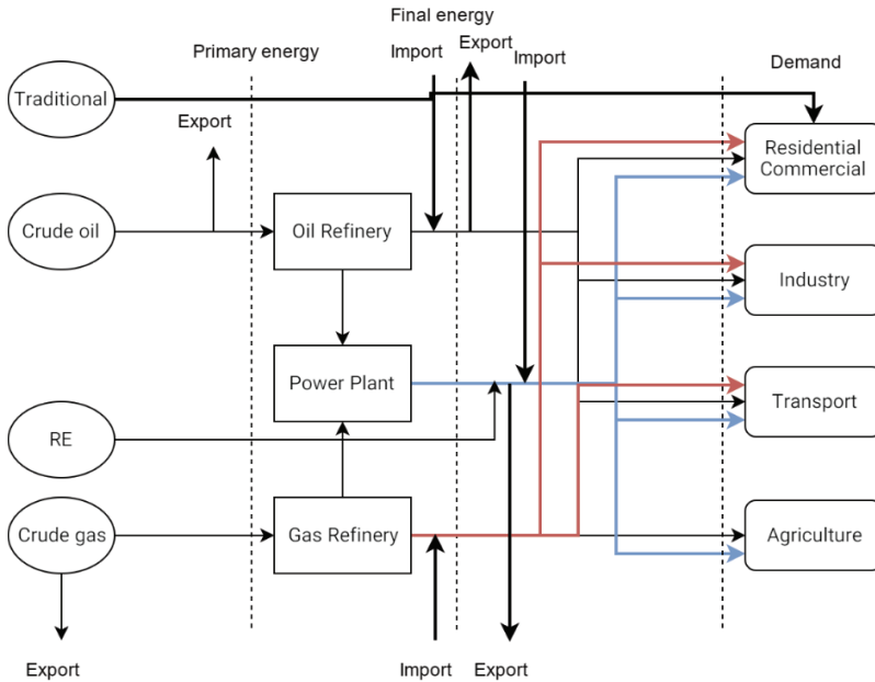
شکل ۲. نمودار مرجع انرژی
